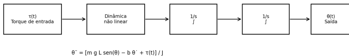
Figura 1 — Representação em blocos da dinâmica do pêndulo invertido.
